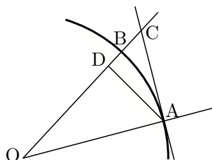
図 3.12 点 O を中心にした半径 1 の円周上に点 A, B をとる。点 A を通る円の接線を引く。それが OB を延長した直線と交わる点を C とする。また、 A から直線 OC に降ろした垂線を AD とする。
