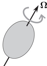
図 6.15 固定された回転軸のまわりを一定のはやさで回転している剛体。回転から右ネジのルールで決まる方向を向き、回転の角速度と同じ大きさをもった角速度ベクトル \Omega によって回転が特徴づけられる。
