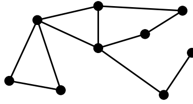
図 7.7 このように、いくつかの頂点を線分で結んだものをグラフと呼ぶ。
