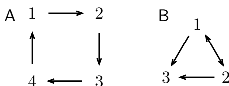
図 7.5 (7.7.1) の行列 A 、(7.7.2) の行列 B から決まる「つながり」の様子。行列の i, j 成分がゼロでないとき j \rightarrow i という「つながり」が作られるとする。行列 A については、任意の二つの数が何本かの矢印を介してつながっているが、 B については、たとえば、3 から 1 へのつながりは作れない。
