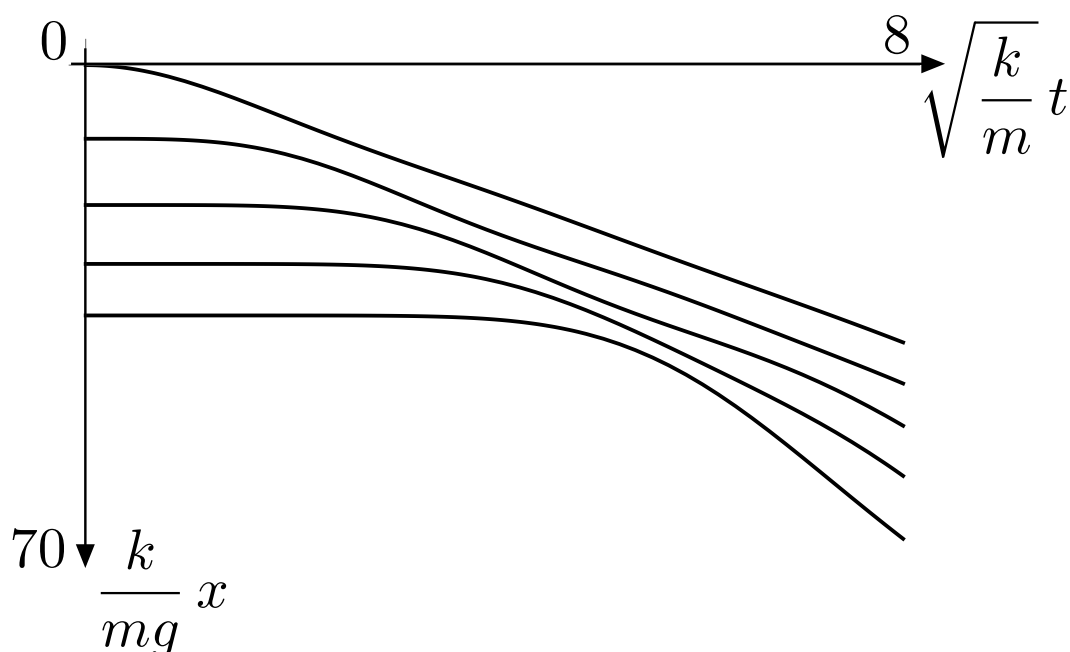
図 5.9 5 個の粒子をつないだ場合の粒子の位置の時間変化。連立常微分方程式 (5.3.108) で N = 5 としたものを数値的に解いて描いた。横軸は時刻、縦軸は位置だが、どちらも無次元量をプロットしている。バネの自然長を \ell_0 = 6mg/k と選んで粒子どうしが衝突しないようにした（これはかなりわざとらしい）。こんな簡単なモデルでも、一番下の粒子は最初のうちはほとんど動かず、上から押されて「手を放したことを教えてもらって慌てて落ち始める」様子が見られる。
