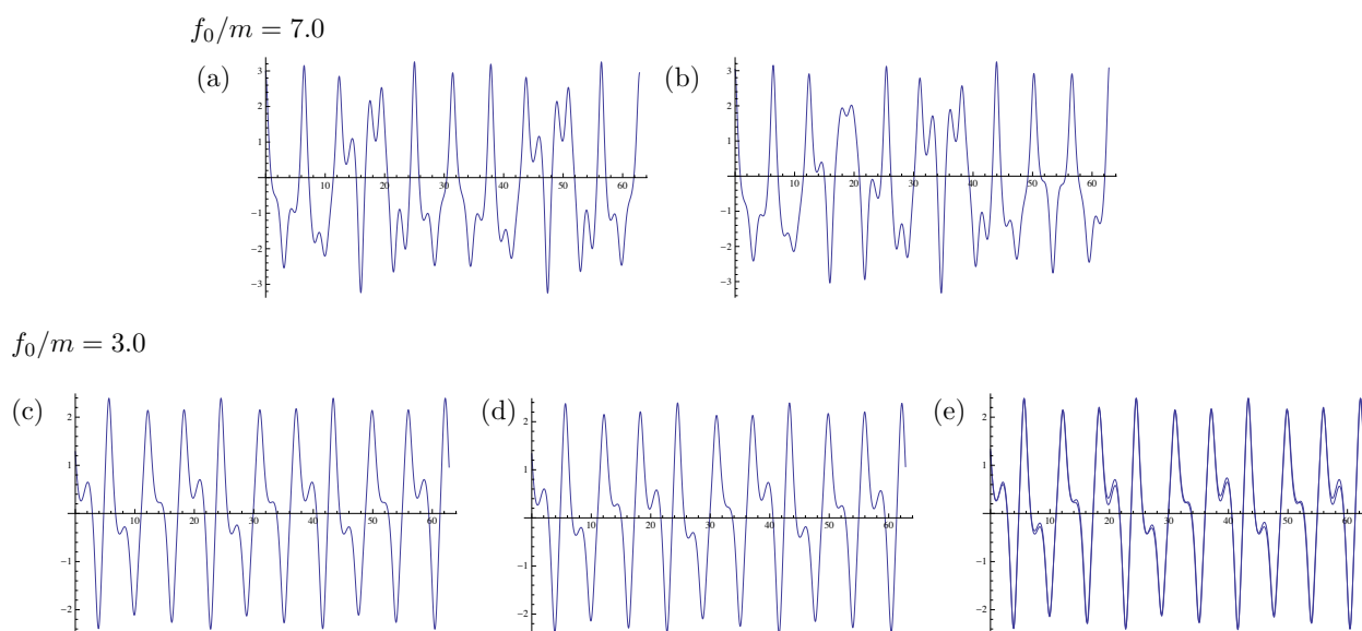
図 5.13 ダフティング方程式 (5.3.110) の解の数値計算の結果。 (a), (b) f_0/m = 7.0 としたカオスの領域で、初期値が 0.05 だけずれた二つの解を描いた。少し時間が経つと、初期値のずれが大きく増幅され、両者のふるまいは似ても似つかなくなる。 (c), (d) f_0/m = 3.0 のときに同様に初期値が 0.05 だけずれた二つの解を描いたが、これでは区別がつかない。二つを重ねて描いた (e) をみると、わずかな相違が残っていることがわかる (しかし、時間がたつとその相違も消えていく)。
