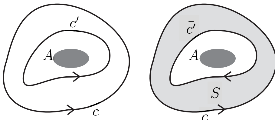
図 10.30 系 10.9 の状況と証明のアイディア。左図の道 c を、領域 A に触れずに、連続的に変形して、道 c' にすることができる。右図では、道 c' の向きを逆転した道 \bar{c}' と道 c を境界にもつような面 S を示した。この面についてストークスの定理を使う。
