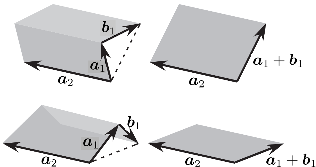
図 7.2 符号付き面積（ディターミナント）が \det[\mathbf{a}_1, \mathbf{a}_2] + \det[\mathbf{b}_1, \mathbf{a}_2] = \det[\mathbf{a}_1 + \mathbf{b}_1, \mathbf{a}_2] を満たすことを幾何的になつとくするための図。式の両辺と左右の図の面積が対応する。上は、 \det[\mathbf{a}_1, \mathbf{a}_2] と \det[\mathbf{b}_1, \mathbf{a}_2] がどちらも正の場合。補助線をにらみながら、平行四辺形の等積変形をおこなえば、左右の二つの図形の面積が等しいことはすぐにわかるだろう。下は、 \det[\mathbf{a}_1, \mathbf{a}_2] が正で \det[\mathbf{b}_1, \mathbf{a}_2] が負の場合。やはり等積変形して、面積の引き算をすると、右側の平行四辺形の面積と一致することがわかる。この例からわかるように、線形性が成り立つためには、単なる面積ではなく、符号付きの面積を考える必要がある。
