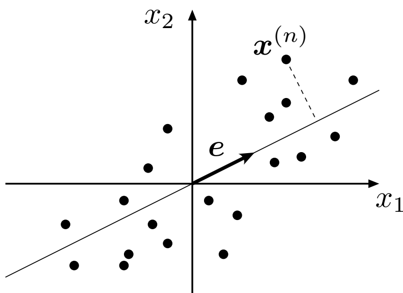
図 7.4 主成分分析の概念図。 d = 2 の場合。2 成分のデータ（例えば、物理と英語のテストの成績）を 2 次元の座標にプロットした（平均値はゼロとする）。原点を通る直線を描き、それに沿った座標を使ってデータを特徴づけることを考える。図のように、データ点が描く図形が「最も伸びている方向」に直線を引けば、最も上手にデータを特徴づけられる。
