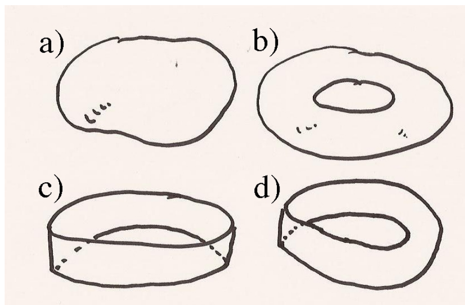
図 10.21 様々な面。a) は、球面を少しいびつにしたような面のつもり。b) は、ドーナツの表面、あるいは浮き輪みたいな図形で、トーラスと呼ばれる。a), b) は境界のない面の例である。(われわれに見えている) 外側を表とよぶ。c) は紙テープの両端を貼り合わせてつくったような輪であり、上下に円周状の境界がある。ここでは、このような境界付きの面も考えている。d) は紙テープを貼り合わせるときに一回ねじってつくったメビウスの帯の図 (のつもり)。この場合は、仮に「表」と決めたところから表面をたどっていくと「裏」に達してしまう。このような「向き付け不可能」な面についてはベクトル場の面積分は定義できない。
