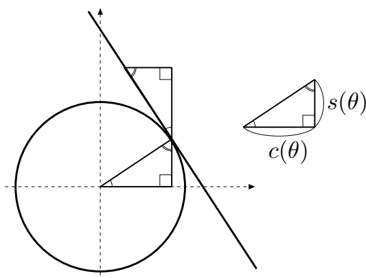
図 3.13 半径 1 の円と円周上の点 (c(\theta), s(\theta)) を通る接線。円の中心と点 (c(\theta), s(\theta)) を結ぶ線分は接線と垂直だから、図の三角形は合同。よって、接線の座標が (3.2.101) で表されることがわかる。ここでは、 c(\theta) > 0, s(\theta) > 0 の場合を描いたが、点が他の象限にあるときにも同様に作図できる。
