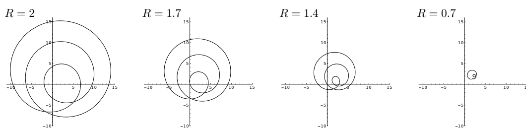
図 2.7 F(x) = x^3 + x^2 + ix + 2 + 2i として、四通りの R の値について、 \theta を 0 から 2\pi まで動かしたときに F(Re^{i\theta}) が描く曲線を図示した。 R が大きい一番左の図では曲線は原点のまわりを 3 回まわっているが、 R が小さい一番右の図では曲線は原点を囲んでいない。これらの途中の R で曲線がちょうど原点を横切る (図には二つの状況を示したが、もう一つ横切る状況がある。これら三つが F(x) = 0 の三つの解に対応する)。
