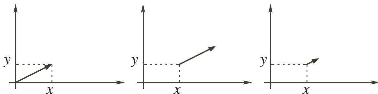
図 10.4 場所 (x, y) において、原点から外向きを向いた単位ベクトルをつくる方法。左の図は、位置 (x, y) を表す位置ベクトルの普通の描き方。原点が始点になっている。ここでベクトルを平行移動して (x, y) を始点にすると、真ん中の図のようになる。さいごに、このベクトルを大きさ \sqrt{x^2 + y^2} で割れば、長さ 1 のベクトルになる。この雰囲気伝えるのが右の図（この図の座標軸は長さの次元をもっている。一方、単位ベクトルの長さは無次元の 1 である。よって、本当のことをいうと、単位ベクトルを図示することにそれほど意味はない）。
