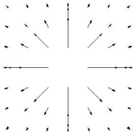
図 10.3 原点にある点電荷のつくる電場の模式図。xy 平面のいくつかの点について、その点における電場ベクトルを、その点を始点とするようなベクトルで表した。図 10.1 と同様、ベクトルの終点に意味はない。電場は原点付近で発散するので、ベクトルはいくらでも長くなってしまう。図を描こうとすると、どうしてもベクトルどうしが重なってしまっ場合が悪い。
