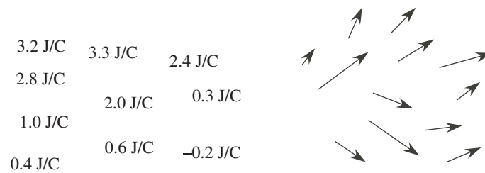
図 10.1 場の気楽なイメージ。スカラー場（左）とは、空間の各点に数字（ただし、単位をついた数字）がびっしりとならんでいるようなもの。ベクトル場（右）とは、空間の各点に矢印がびっしりとならんでいるようなものだ。ただし、これは位置ベクトルではないので、矢印の終点にはさしたる意味はない。矢印の始点の場所に、この矢印で表されるようなベクトルが「乗っかっている」とイメージしよう。矢印の向きはベクトルの向きに等しく、矢印の長さはベクトルの大きさに比例するように描く。なお、いずれの場合も、実際の空間は三次元。さらに、図には何も描いていない隙間の点にもびっしりと数や矢印が乗っていることに注意。
